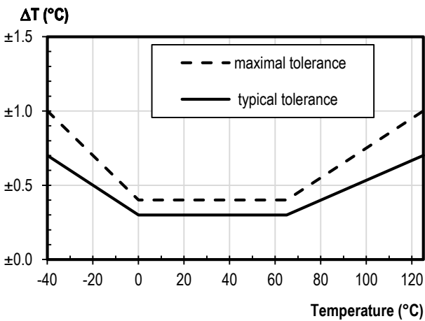
SHT30
