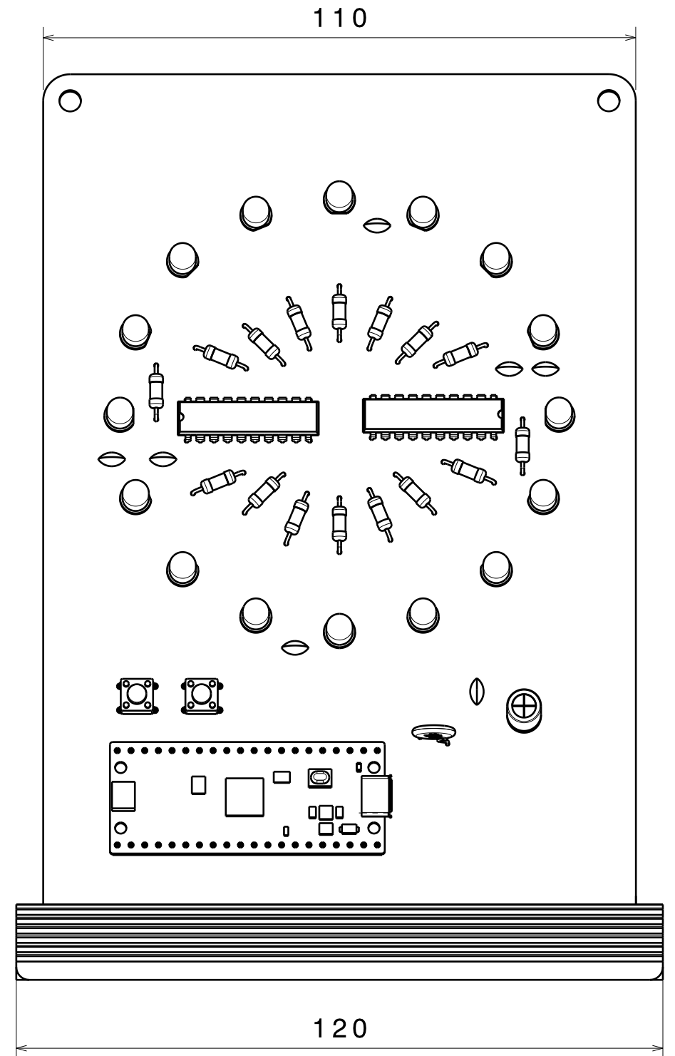
Front view Scale: 1:1
