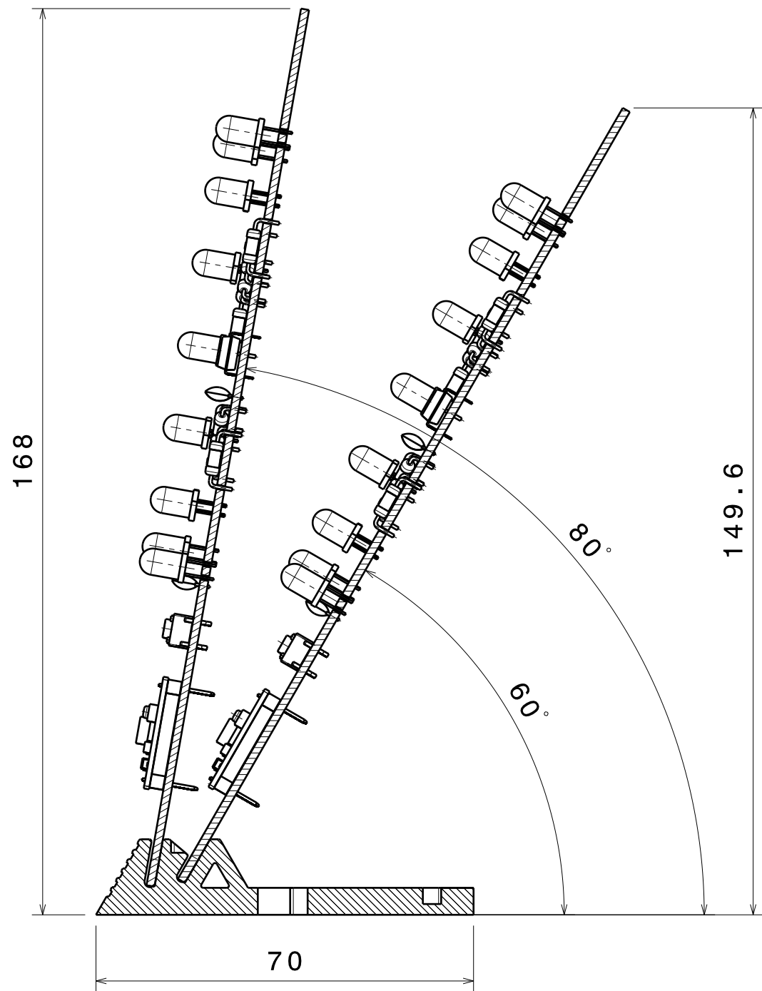
Section view A-A Scale: 1:1
