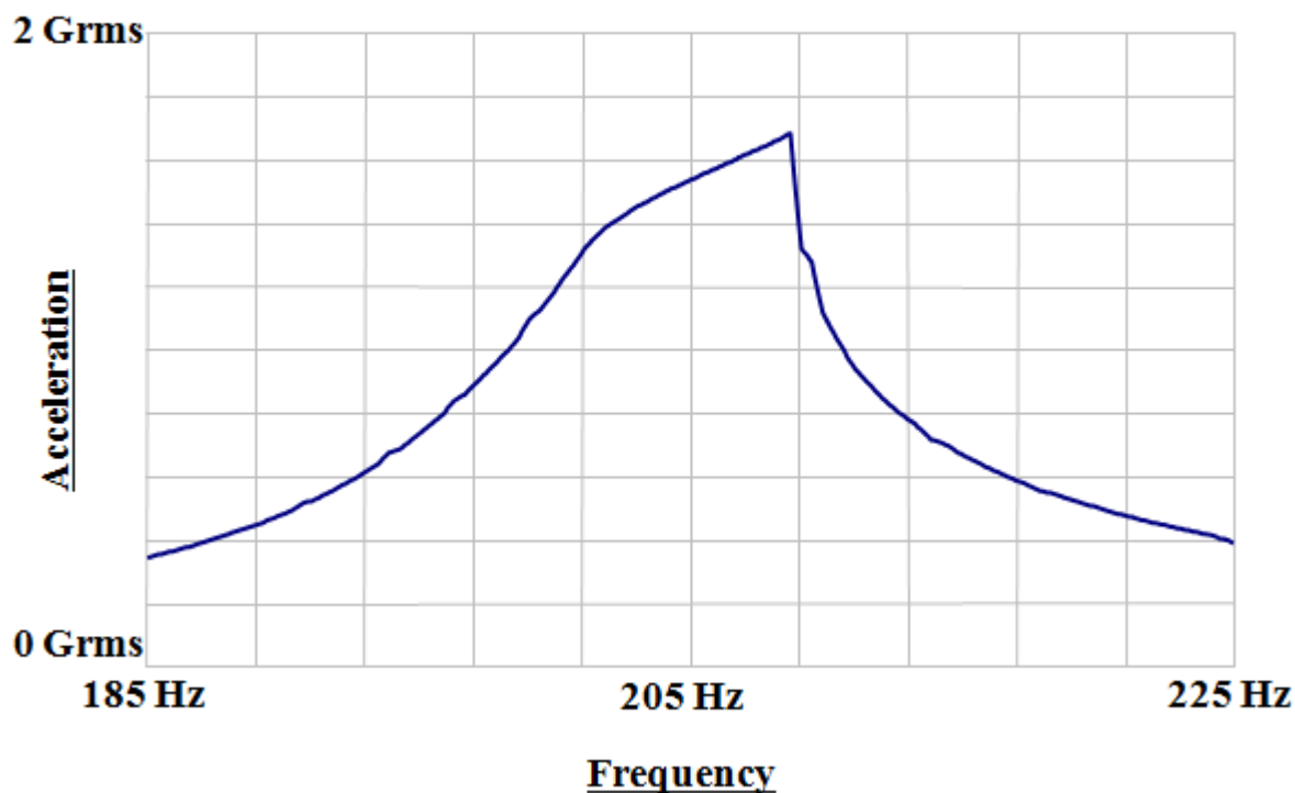
Graph 1. Linear Vibrator Frequency Characteristics / 주파수 특성
