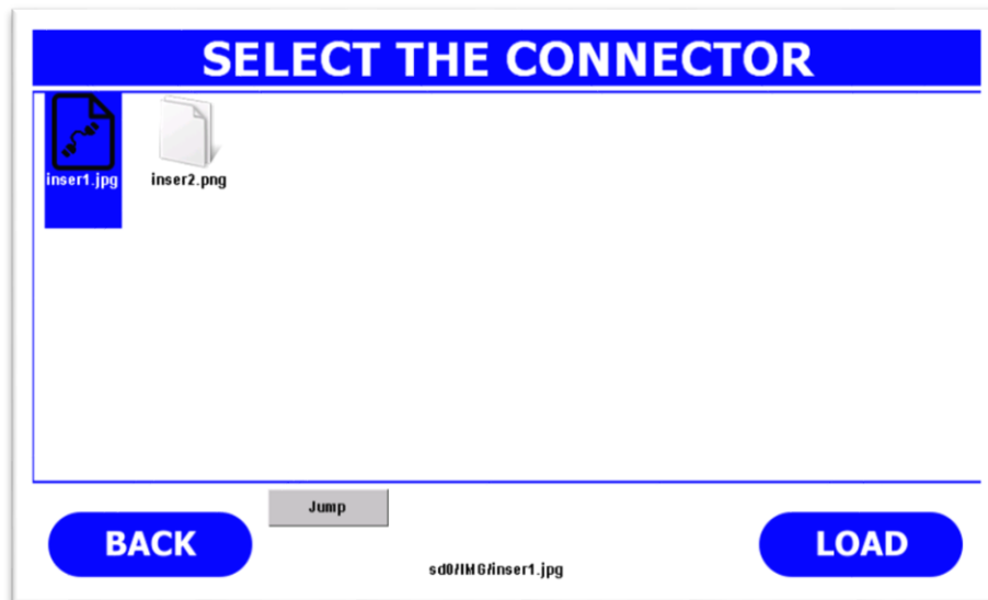
Image 6.- Connector menu.
