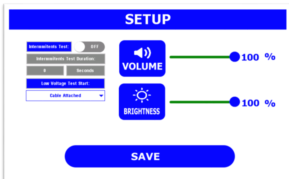
Image 6.- Setup menu.
