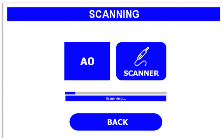
Image 5.- Scanning menu.
