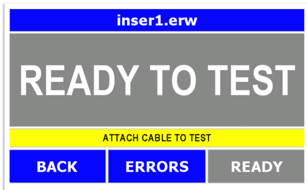
Image 13.- Test menu
