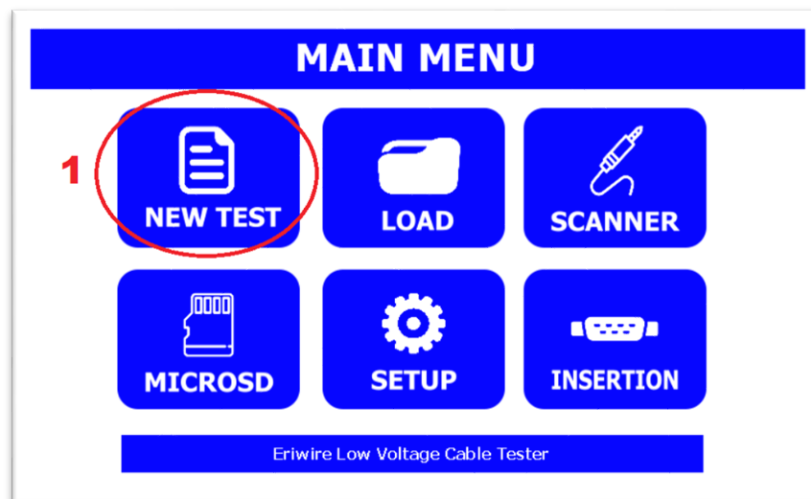
Image 8. -Main menu.
