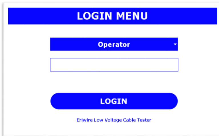
Image 1.- Login Screen.
