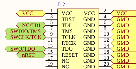
2x10 2.54mm
