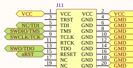
2x10 1.27mm
