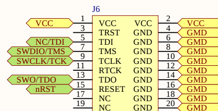
2x10 2.54mm, Edge connector
